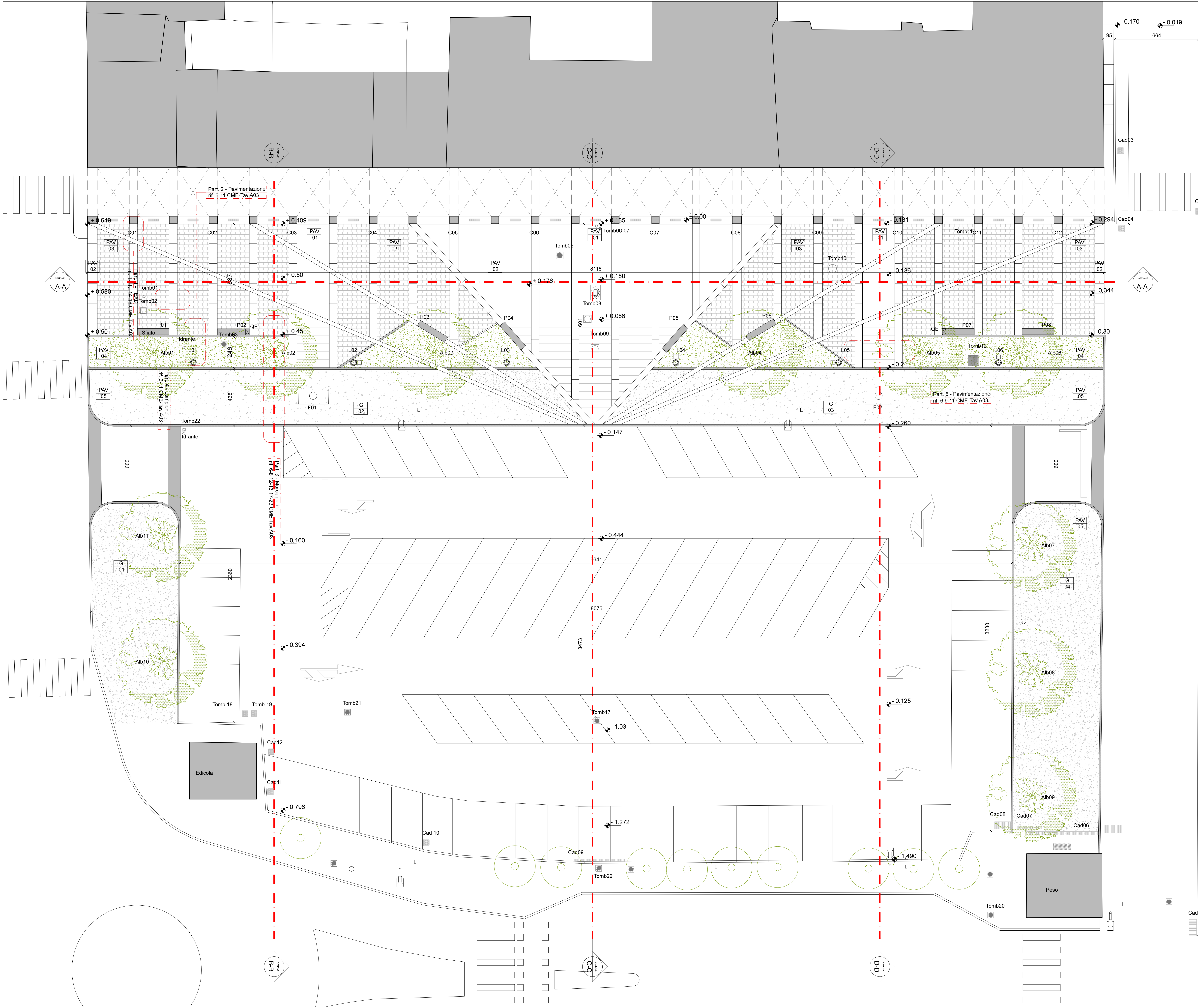
planimetria generale scala 1:500
